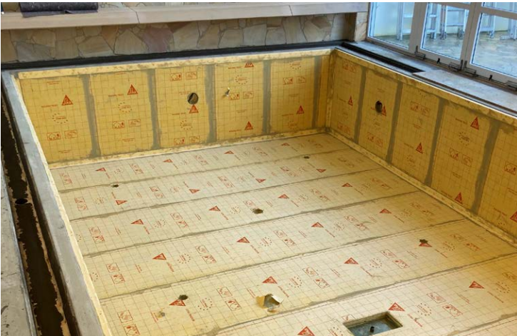
PRODUCT SPOTLIGHT: SikaCeram® Sealing Membrane A & Sika® SealTape F سيكا سيرام سيلين ممبراين / سیکا سيل أف - اغشية عزل مائي للمسبح من الداخل
